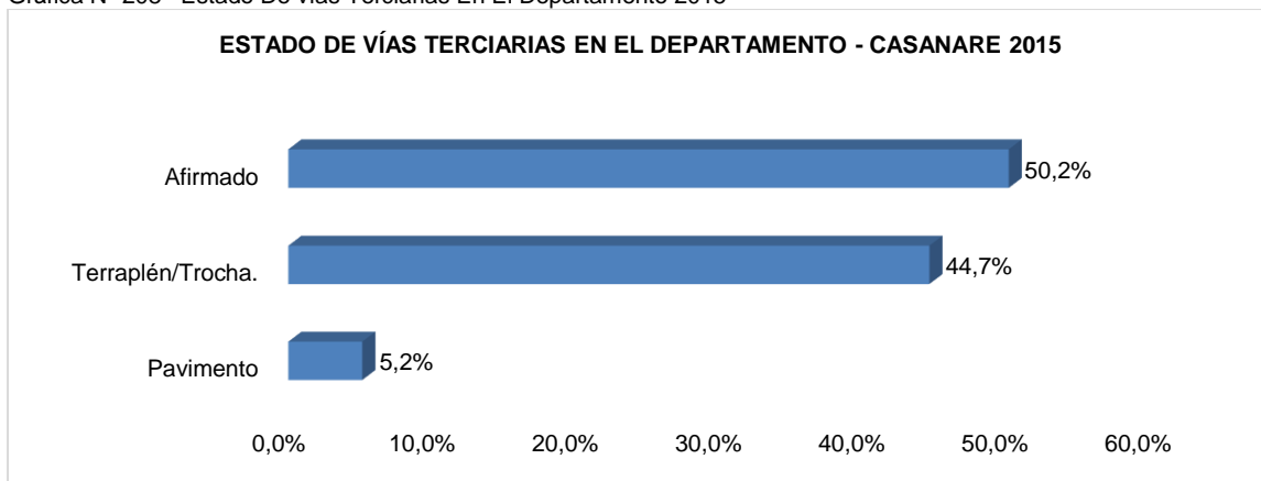
Gráfica N° 208 Estado De vías Terciarias En El Departamento 2015
