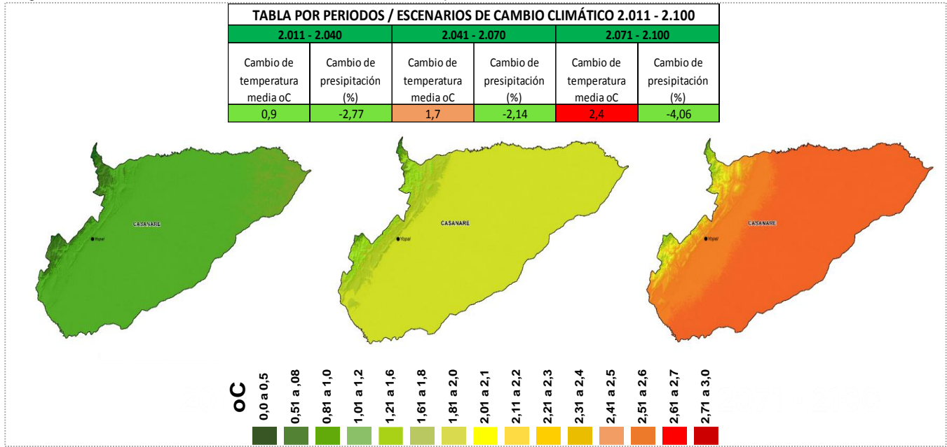
Imagen No.30. Escenarios de Cambio Climático en la variable temperatura
